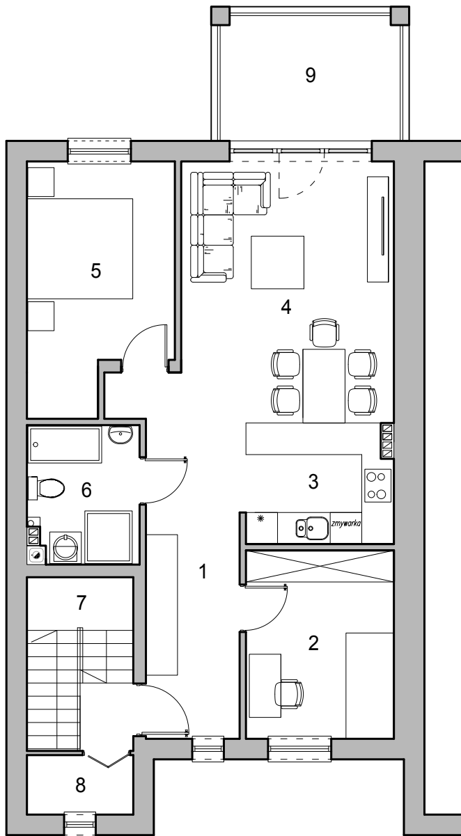
RZUT PIĘTRA BUDYNEK NR 1
