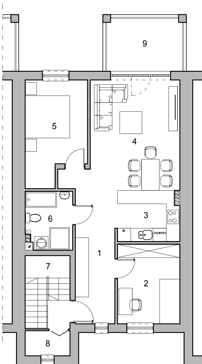
RZUT PIĘTRA BUDYNEK NR 2
