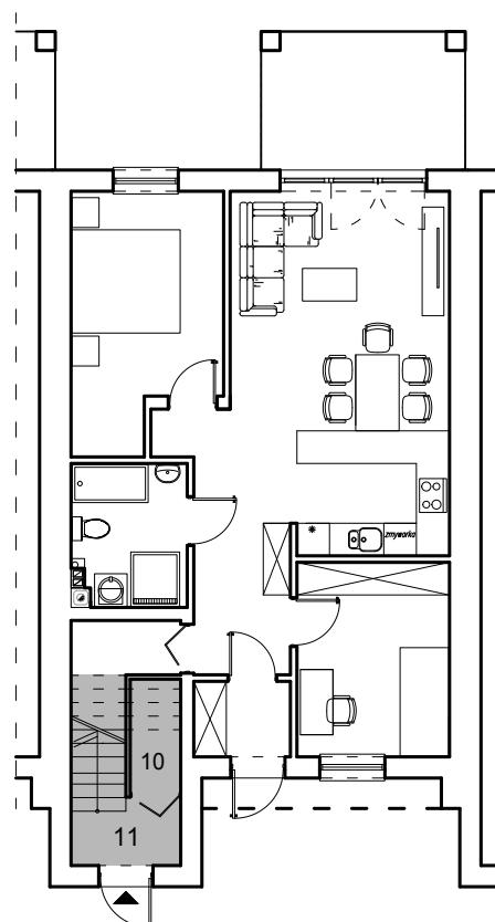
RZUT PARTERU BUDYNEK NR 6
