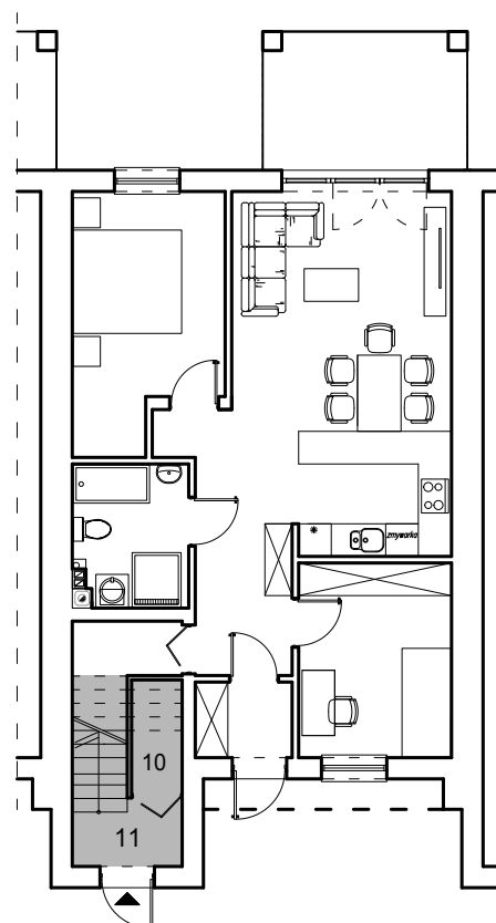
RZUT PARTERU BUDYNEK NR 7
