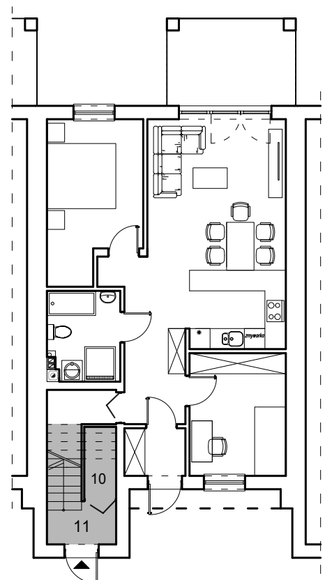
RZUT PARTERU BUDYNEK NR 8
