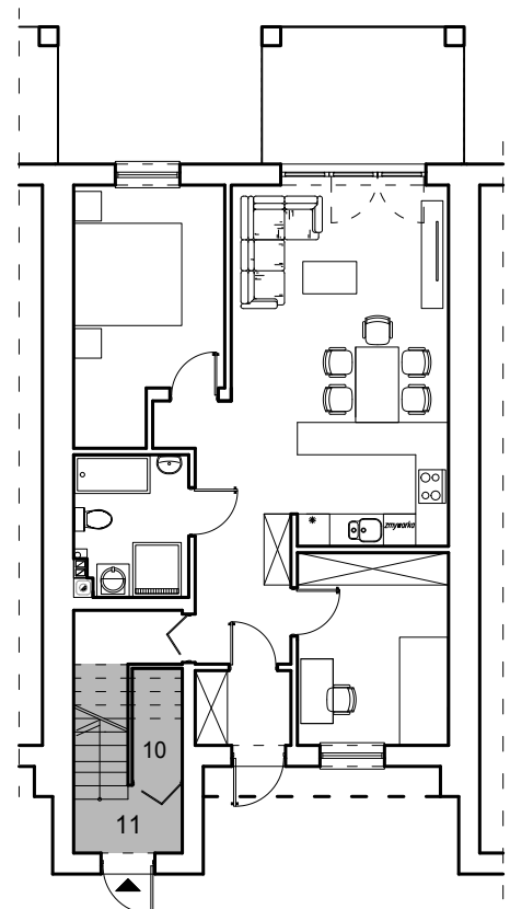
RZUT PARTERU BUDYNEK NR 9
