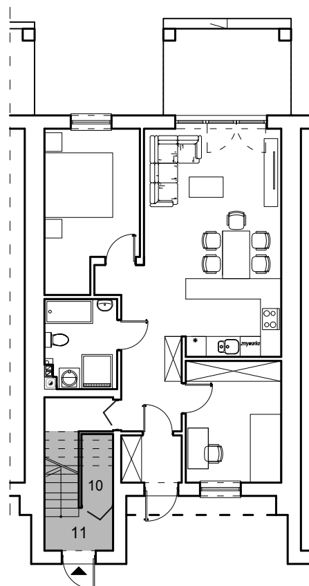
RZUT PARTERU BUDYNEK NR 11
